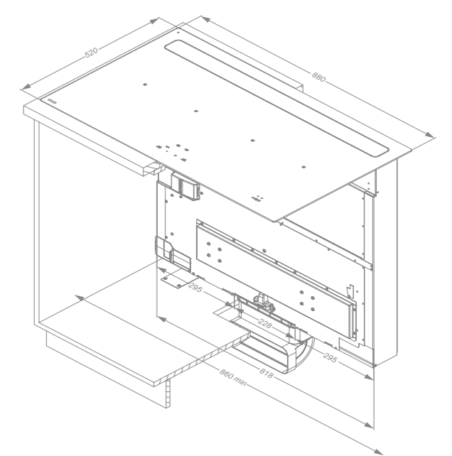
3D tekening
