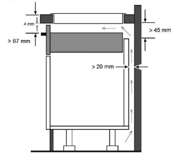
Zijaanzicht
