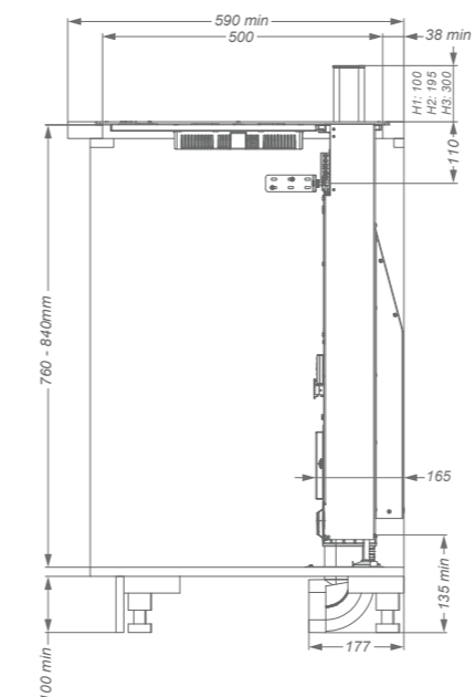
Zijaanzicht
