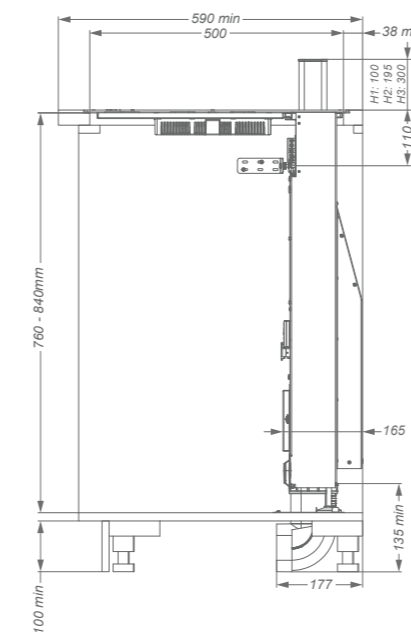
Zijaanzicht
