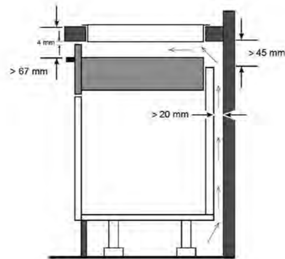
Zijaanzicht
