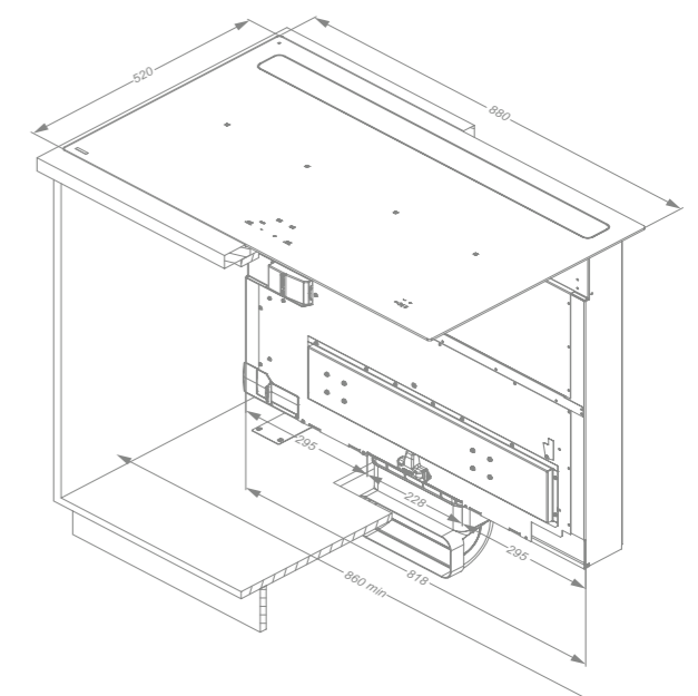
3D tekening
